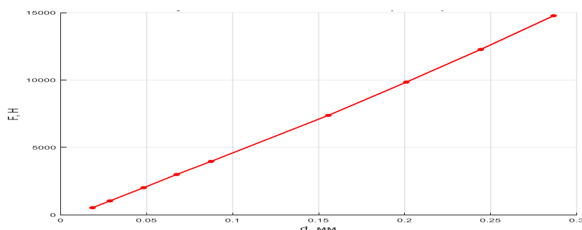
Рисунок 2 - Зависимость глубины вдавливания от приложенной силы при проведении испытаний
