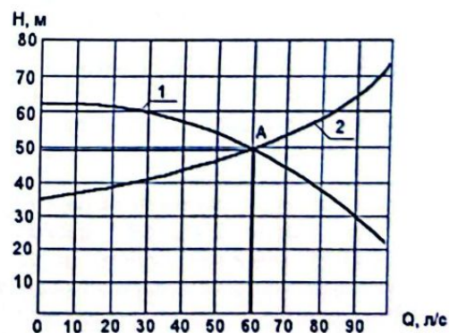
Рисунок 1. Совмещение характеристик насоса и водопроводной сети
