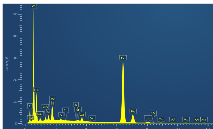
Рисунок 4 - Спектр ГБФ 2, уч.1
