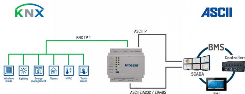
Рис. 2. Система KNX
