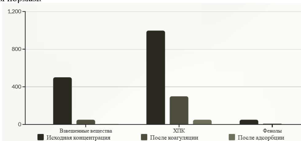
Рис 3. Эффективности методов коагуляции и адсорбции
