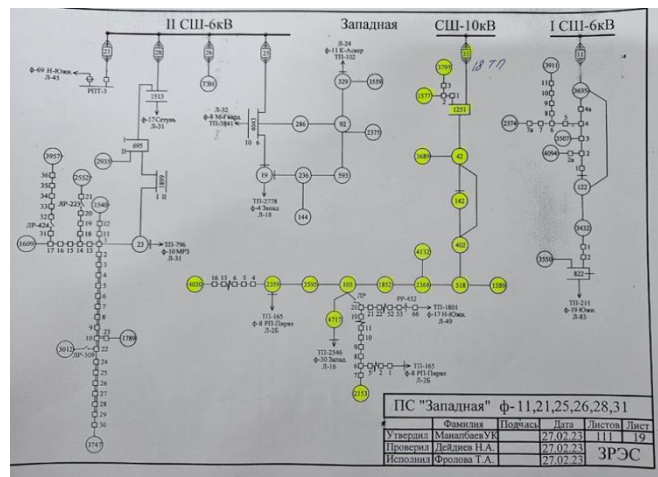
Рис. 2. Схема электрической сети 10кВ фидера №31 ПС «Западная» г. Бишкек.
