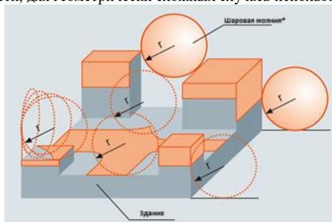
Рис. 2. Схематическое применение метода шаровой молнии к зданию с сильно изрезанной поверхностью
