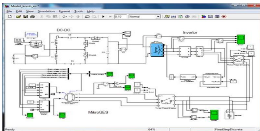
Рисунок 3. Компьютерная модель комбинированного автономного источника энергии на базе микрогидроэлектростанции и фотоэлектрической солнечной электростанции
