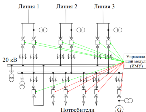
Рис. 4. Типовая схема универсального узла нагрузки (распределительного пункта РП 20 кВ)
