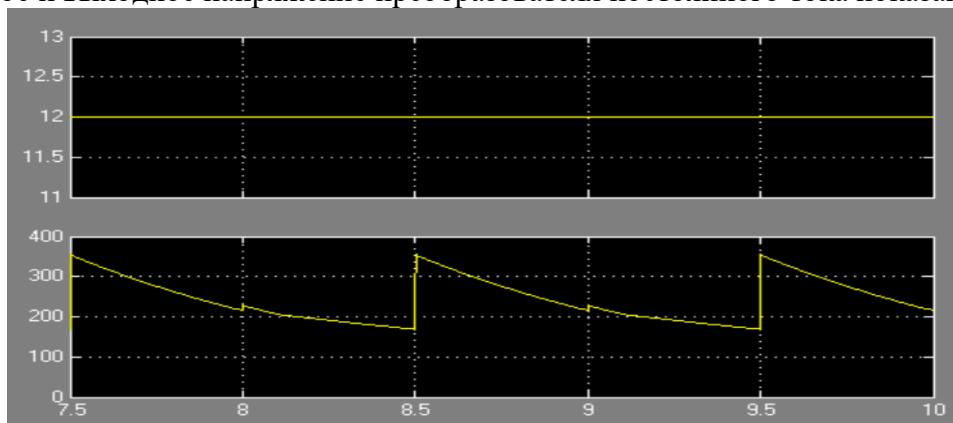
Рис. 4. Входное и выходное напряжение преобразователя постоянного тока в постоянный
