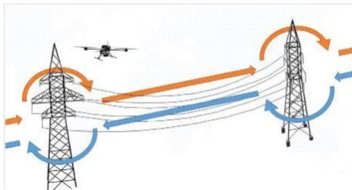
Рис.6. Схема мониторинга ЛЭП с помощью БАС мультироторного типа
