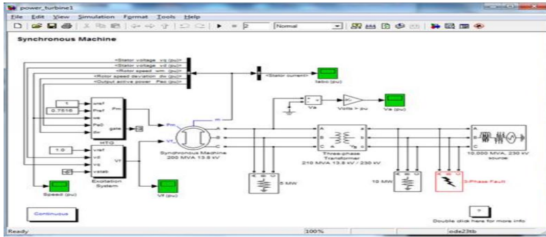
Рис. 1. Компьютерная модель микрогидроэлектростанции
