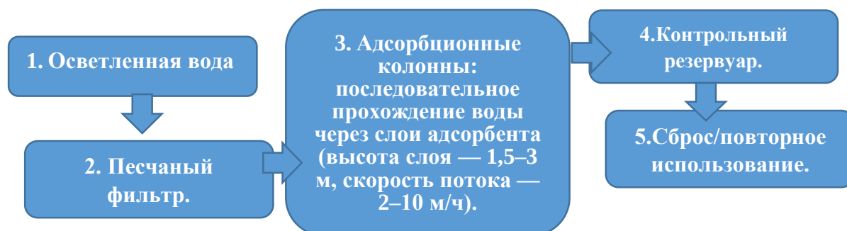
Рисунок 2. Технологическая схема адсорбции.
