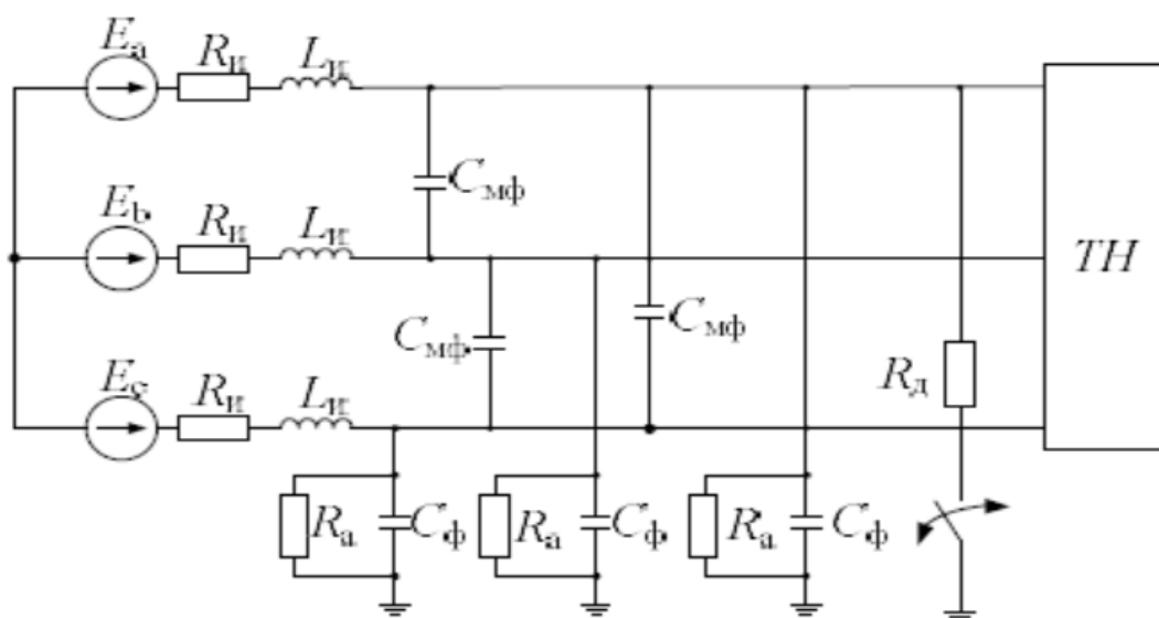
Рис. 1. Расчетная схема исследуемой сети в режиме ОДЗ
