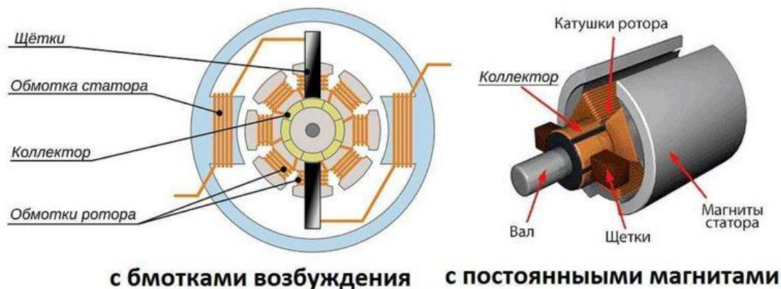
Рис. 4. Конструкция микроэлектродвигателя.
