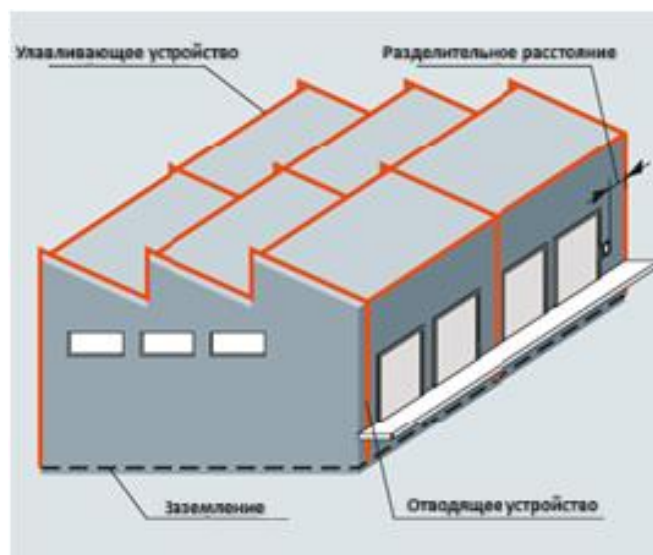
Рис. 1. Система молниезащиты – внешняя молниезащита
