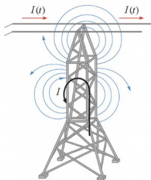
Рис. 1. Схема индукции тока в металлической опоре
