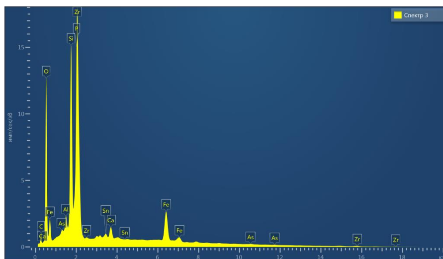
Рисунок 8 - Спектр СМФ 3, уч.3.
