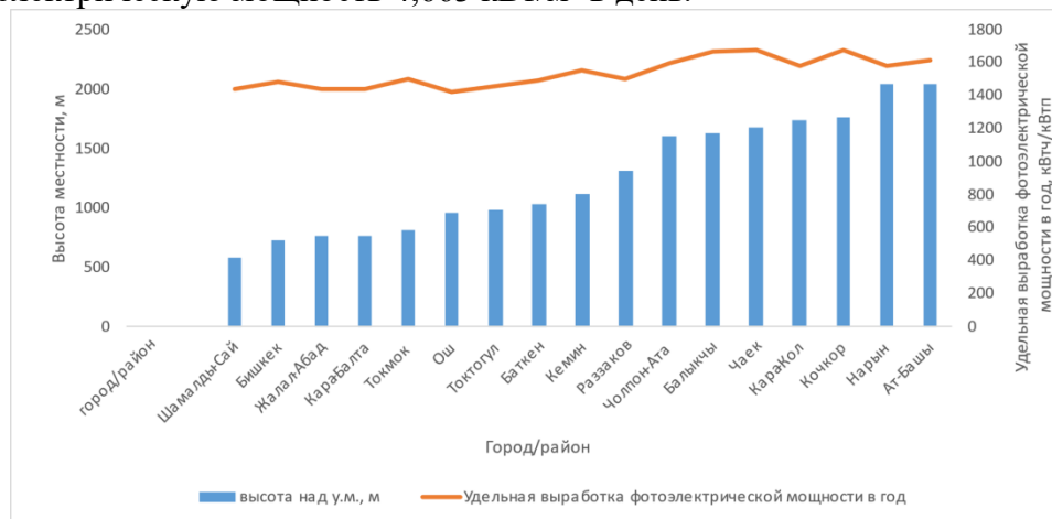
Рис. 2. Зависимость удельной выработки фотоэлектрической мощности за год от высоты местности.
