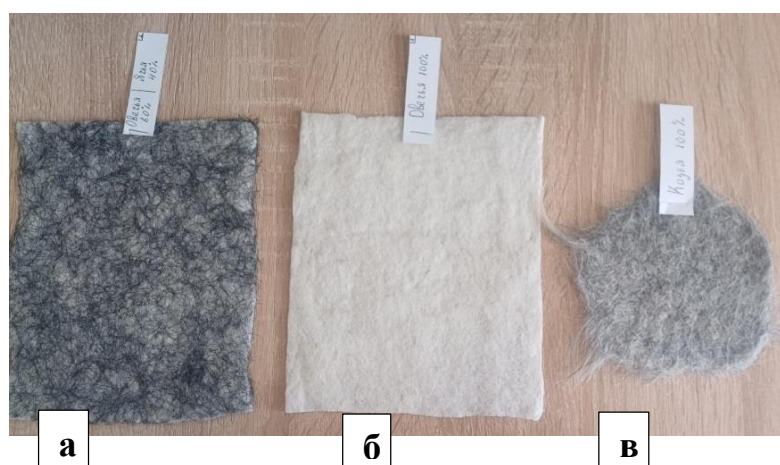
Рис. 1 Экспериментальные образцы - а) Овечья шерсть 60% / шерсть яка 40% б) Овечья шерсть 100% в) Козья шерсть 100%
