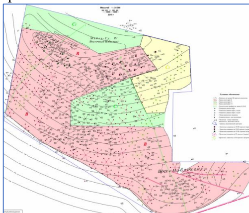
Рисунок 2: Структурная карта с указанием категорий запасов III горизонта нефтегазового месторождения Майли-Су IV – Восточный Избаскент.
