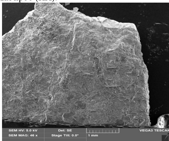
Рисунок 9 - Морфологическая структура крупных частиц ИХ 5X5 мм
