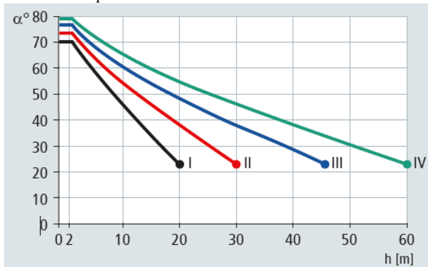
Рис. 3. Метод защитного угла в соответствии со стандартом DIN EN 62305-3
