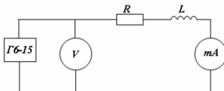
Рис. 2. Схема замещения катушки индуктивности
