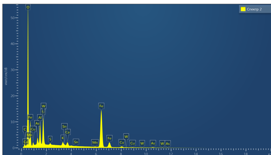
Рисунок 5 – Спектр ГБФ 2, уч.
