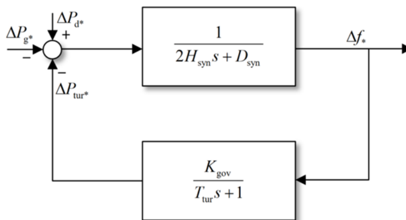
Рис.1. Модель микросети, включающей ветрогенераторы
