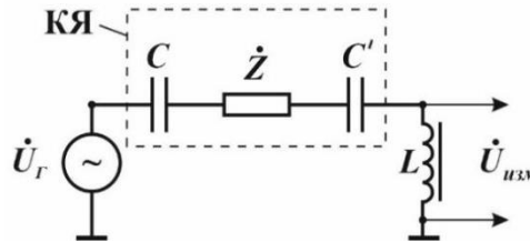
Рис. 2. Электрическая схема замещения устройства оперативного контроля параметров изолированных проводов
