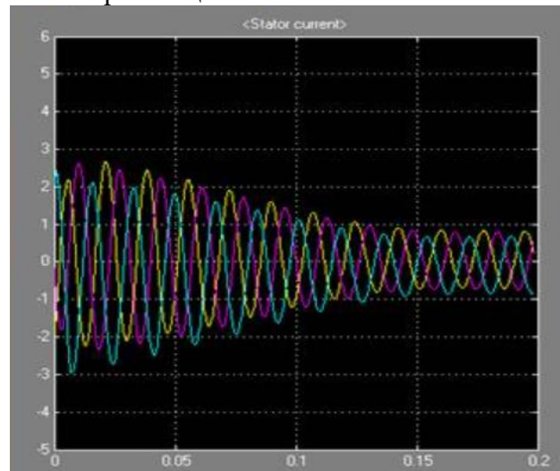
Рис. 2. Осциллограммы изменения тока статора.
