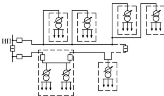
Рис. 1. Общая структурная схема распределительной сети
