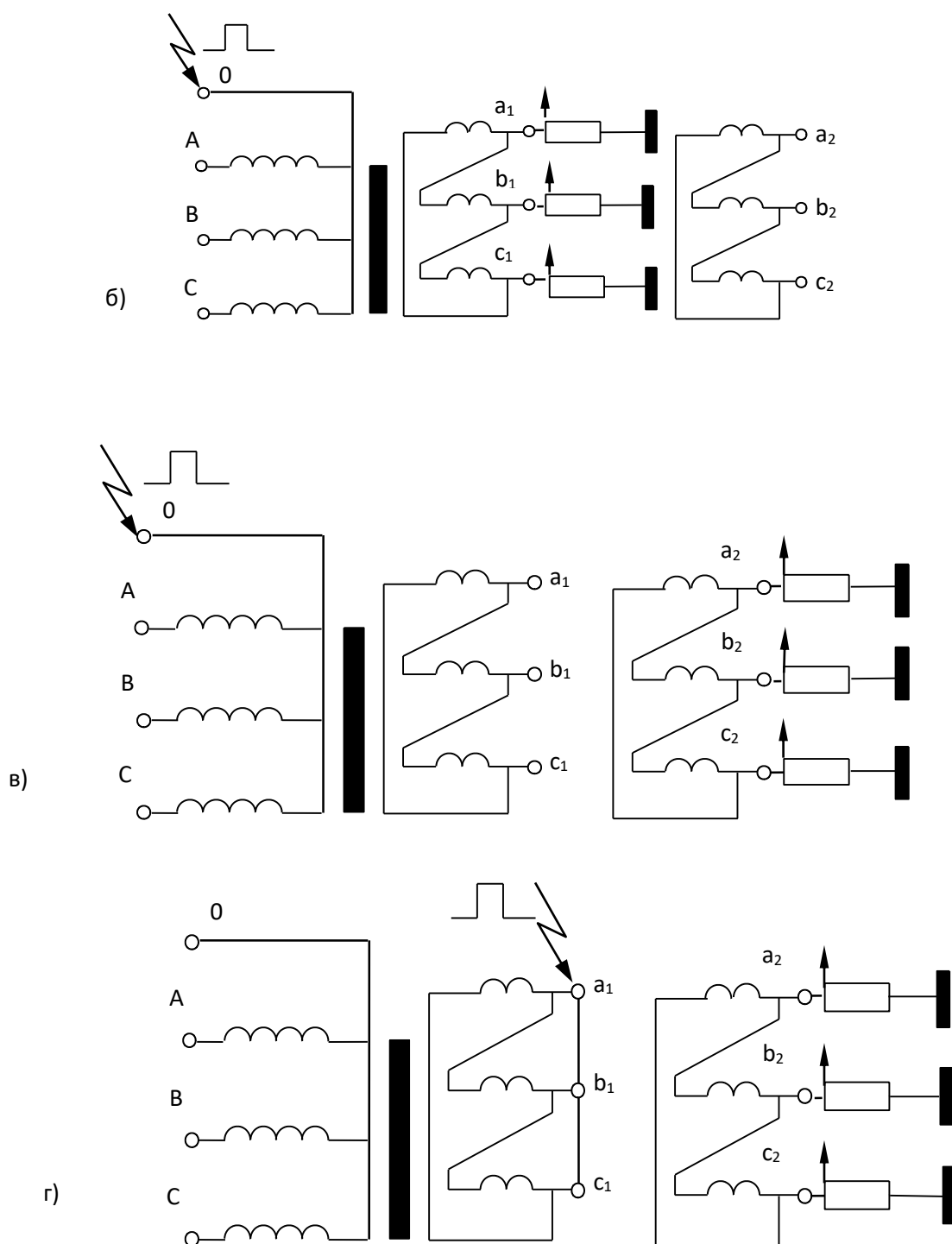
Сүр. 2. - Т-2 трансформаторунун ТВИ ыкмасы менен дефекттерди аныктоо схемалары.
