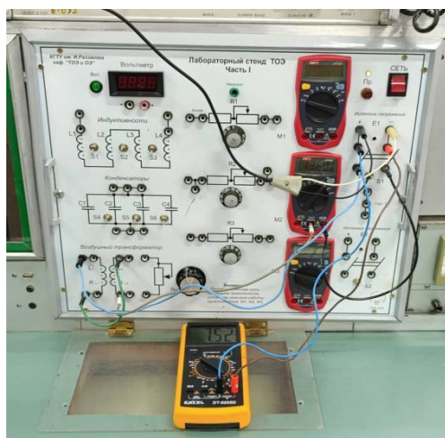
Рис. 3. Экспериментальная лабораторная установка и схема замещения последовательно соединенных катушек индуктивности
