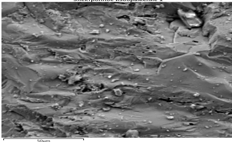
Рисунок 6- Изображение СМФ 1, уч.1. (поверхность основных частиц зона 150 мкм)
