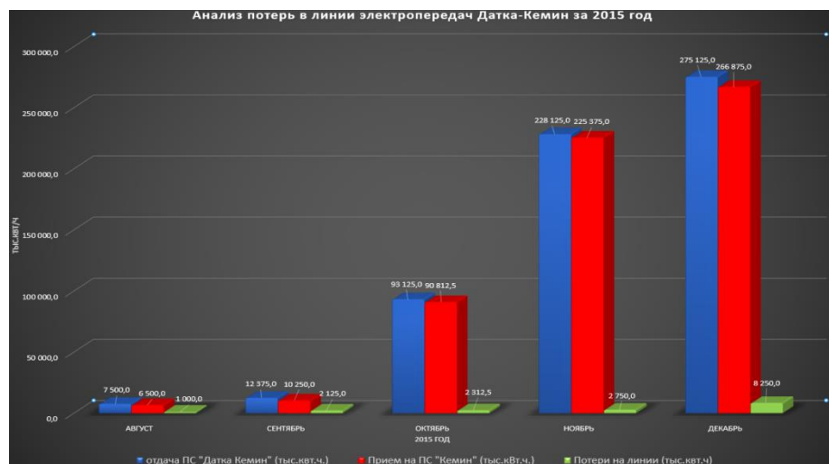
Рис.1. Гистограмма анализа потерь в ЛЭП «Датка-Кемин» за 2015 год.
