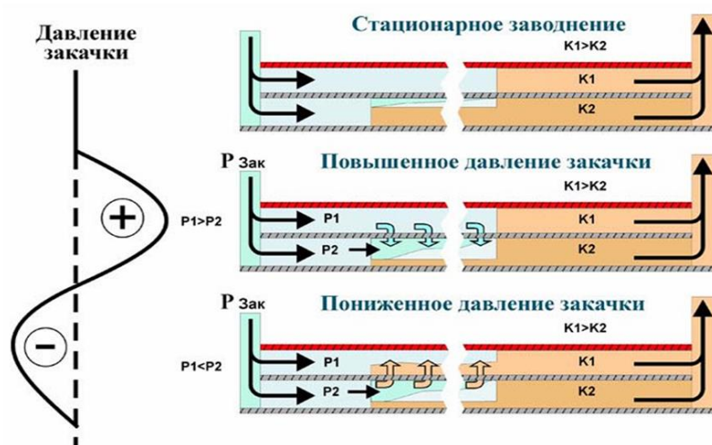
Рисунок 3. Схема циклического заводнения залежи
