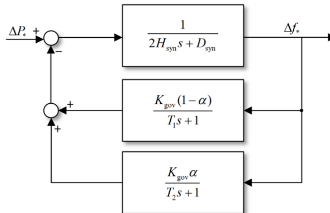
Рис. 3. Модель микросети, содержащей два типа источников энергии
