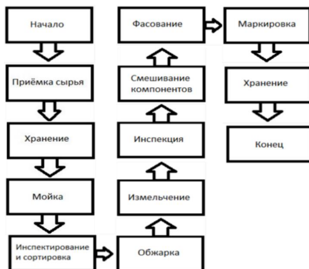
Рис 1. Технологическая схема производства фисташковой пасты
