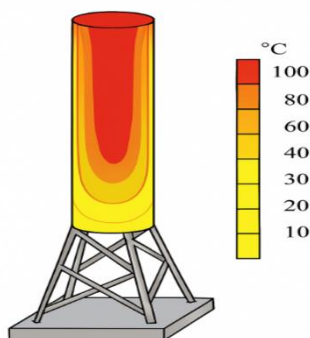
Рис. 2. Температурное распределение по поверхности опоры
