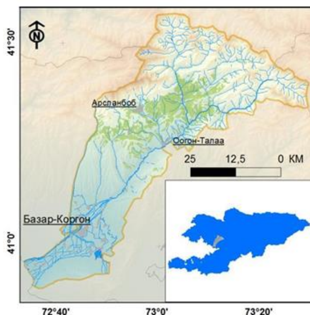
Рисунок 1. Карта расположения селеопасного бассейна реки Кара-Ункур
