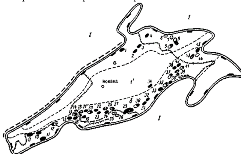
Рисунок 1. Карта-схема Ферганской нефтегазоносной области
