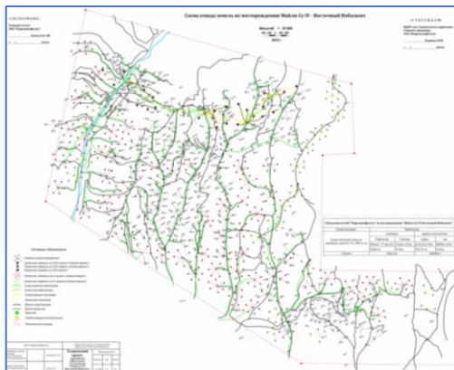
Рисунок 1. Карта схема отвода Земель под месторождение Майли-Су IV – Восточный Избаскент.
