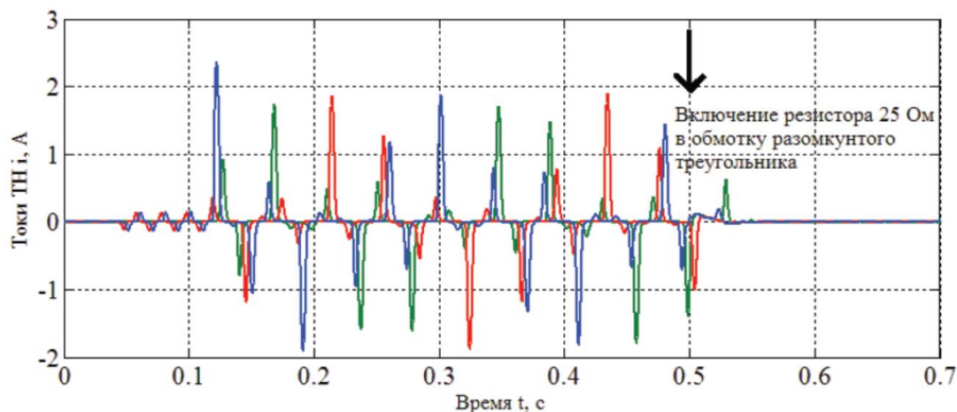
Рис. 3. Расчетные кривые токов в обмотке ВН при подавлении феррорезонанса установкой резистора 25 Ом в обмотку разомкнутого треугольника. C_{\phi}=0,5 \text{ мкФ}
