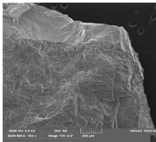
Рисунок 9 - Морфологическая структура крупных частиц ИХ 5X5 мм
