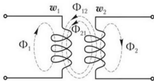
Рис.1. Схема замещения индуктивно связанных катушек
