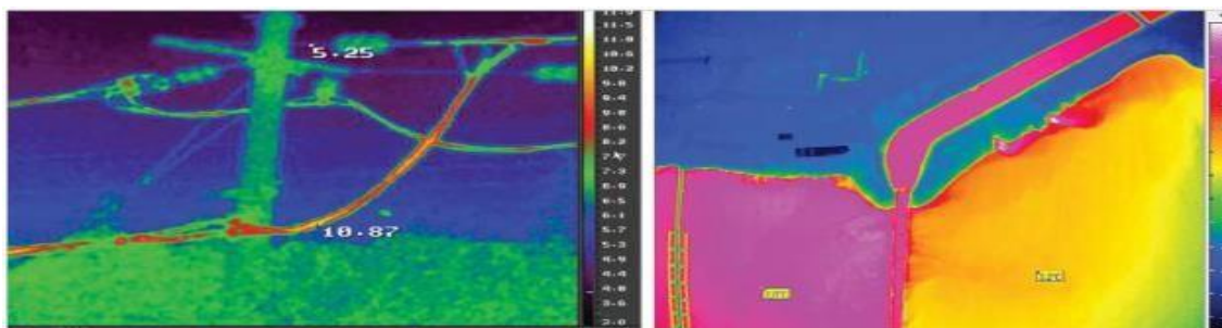
Рис. 7. Пример изображения, полученного при ИК съемке тепловизором: с земли (слева), с БАС Птеро G0 (справа)
