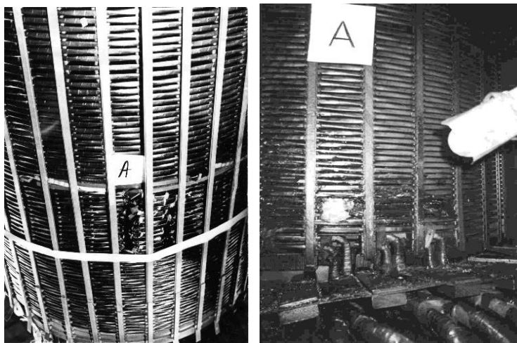
Сүр. 1. ТДЦ-250000/220 трансформаторунун ТЧ оромунда витоктун кыска туташуусунун пайда болушунун мисалы.
