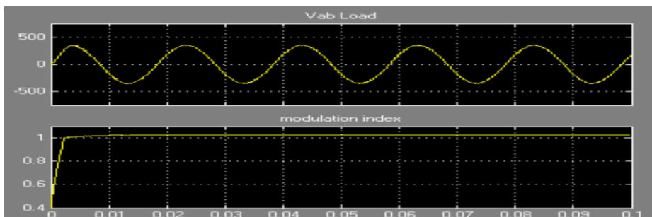
Рис. 5. Осциллограммы инвертора
