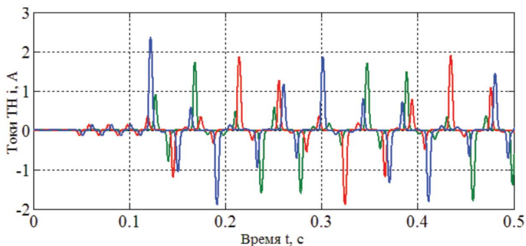
Рис. 2. Расчетные кривые токов в обмотке ВН при феррорезонансе, возникшем в результате отключения ОЗЗ. C_{\phi} = 0,5 \text{ мкФ}
