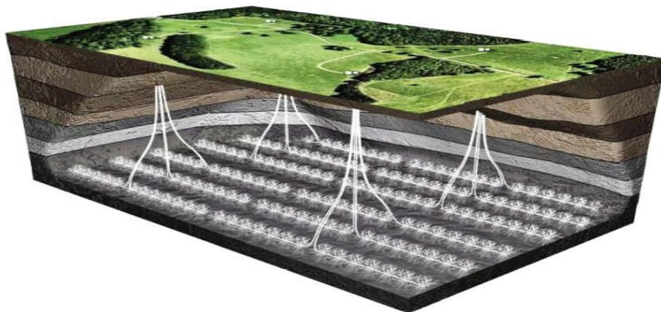
Рисунок 1. Суперскважина – это многокустовая, многозабойная скважина с многостадийным ГРП [1-10].
