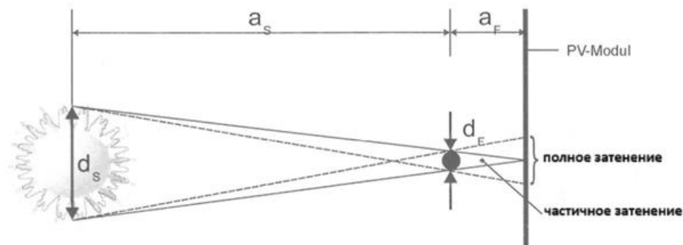
Рис. 4. Минимальное расстояние между опорой и опорой Улавливающего устройства и фотоэлектрического модуля для предотвращения затенения сердечника.
