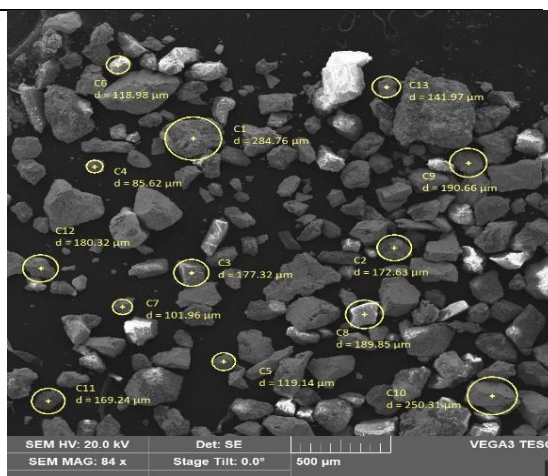
Рисунок 11 – Диаметр основных частиц СМФ (уср.) (Ø 167,7 мкм)
