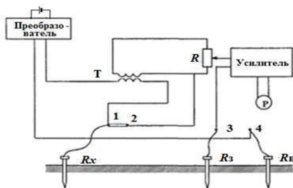
Рис. 1. Структурная схема прибора Ф-4301-М1
