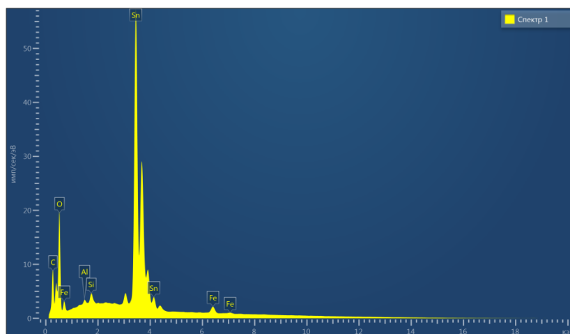
Рисунок 7 – Спектр СМФ 1, уч.1.
