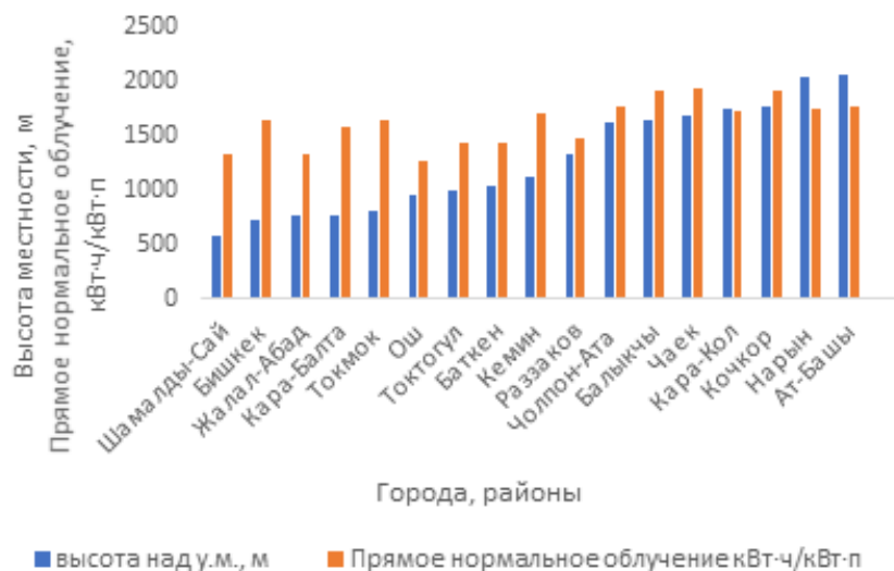
Рис. 3. Зависимость прямого нормального облучения от высоты местности.
