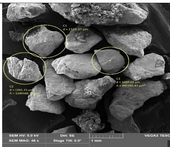
Рисунок 10 –Образец ГБФ (порошкообразный Ø частиц 1-1,5 мкм)
