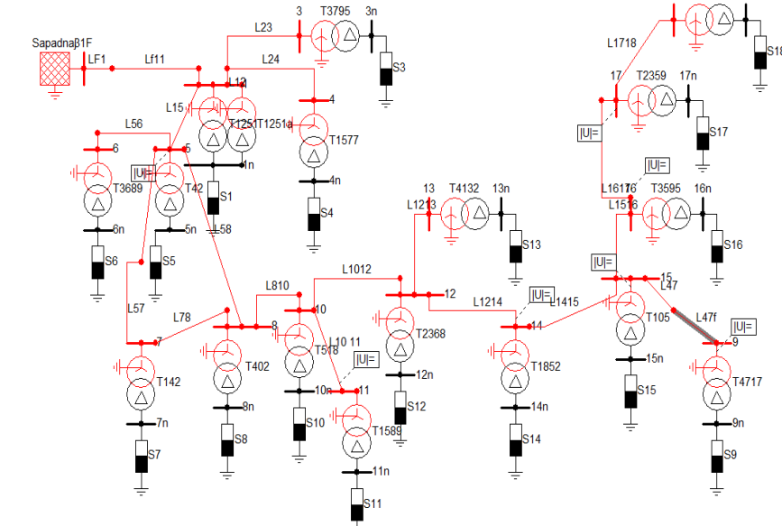
Рис.3. Расчетная схема электрической сети
