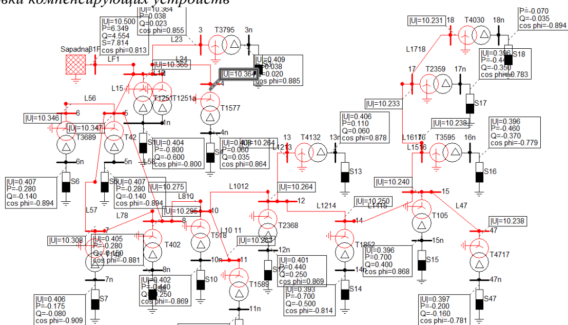
Рис. 4. Результаты расчета Потери мощности в сети
