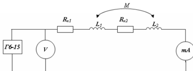
Рис. 3. Экспериментальная лабораторная установка и схема замещения последовательно соединенных катушек индуктивности
