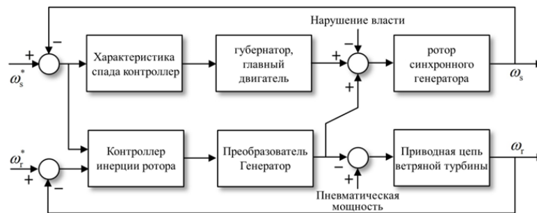
Рис. 4. Модель системы регулирования скорости
