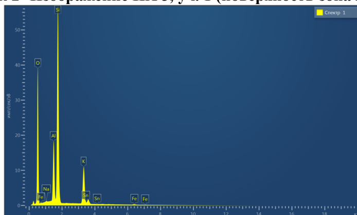
Рисунок 2- Изображение ИХ 3, уч. 1 (поверхность зона 200 мкм)
