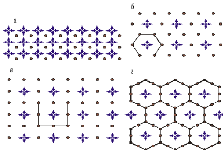
Рис. 1. Системы разработки с площадным заводнением
