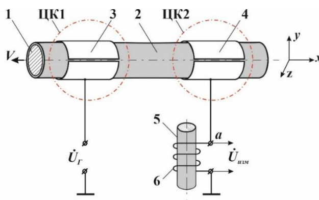
Рис. 1. Принципиальная конструктивная реализация устройства оперативного контроля параметров изолированных проводов
