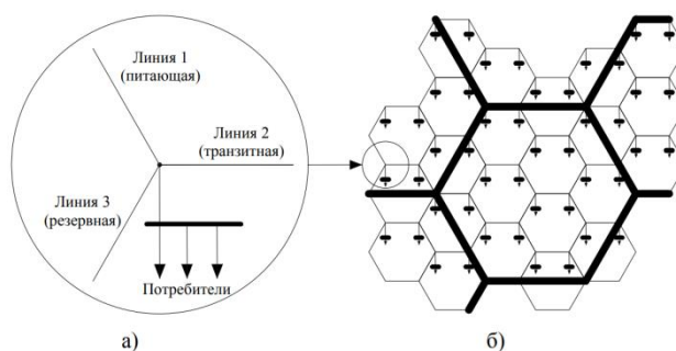
Рис. 3. Принцип формирования распределительной сети и узлов нагрузки С технико-экономической точки зрения основными преимуществами предложенной в работе [5] гексагональной сети являются:
