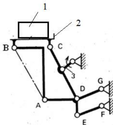
Рисунок 2 – Схема механизма перегрузчика: 1 – заготовки, 2 – площадка с заготовками, 3 – кривошип.
