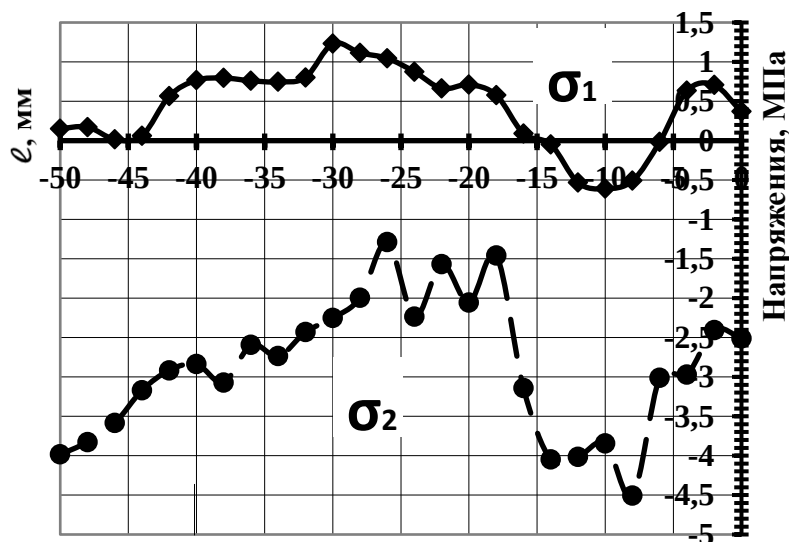
Рисунок 4 - Эпюры главных нормальных напряжений по горизонтальному сечению на левом борту карьера
