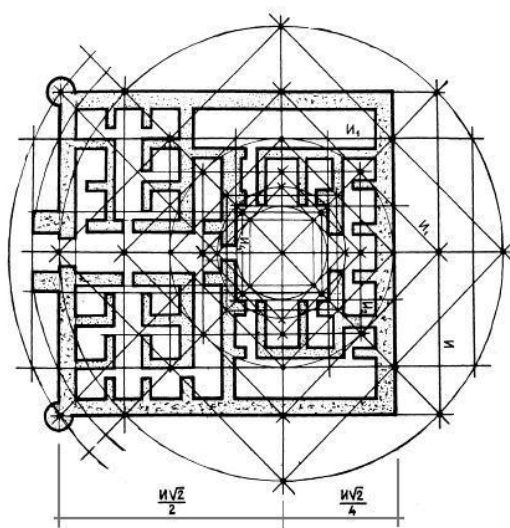
Рисунок 4 – Анализ геометрического построения плана [12]
