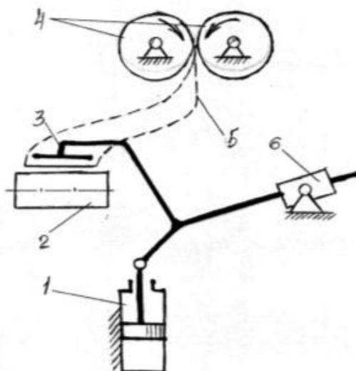
Рисунок 5 – Схема механизма, подающего лист бумаги
