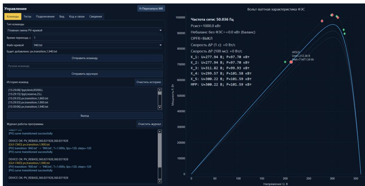
Рисунок 4 - Интерактивный экран визуализации процесса регулирования операционной точки напряжения
