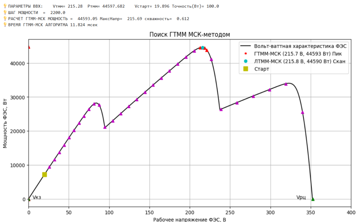
Рисунок 8 – Траектория управления РММ-шаблон 4 с использованием контроллера ГТММ-МСК в Micro-Python
