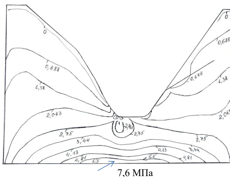
Рисунок 2 - Изолинии распределения максимальных касательных напряжений в модели под влиянием крутопадающего разлома
