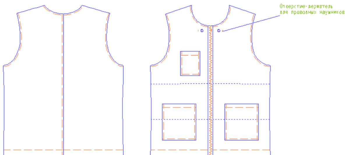
Рисунок 4 – Технический рисунок жилета
