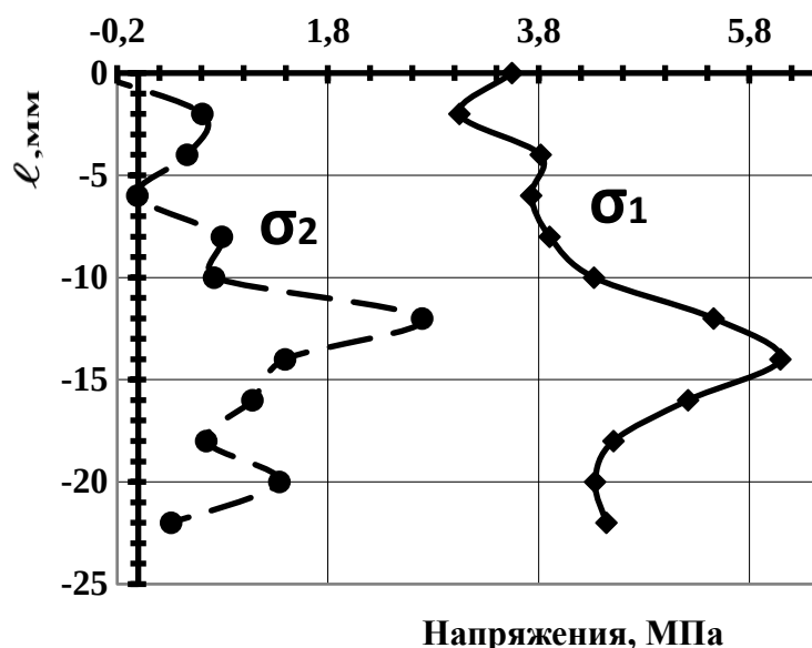
Рисунок 5 - Эпюры главных нормальных напряжений в модели по вертикальному сечению вблизи дна карьера
