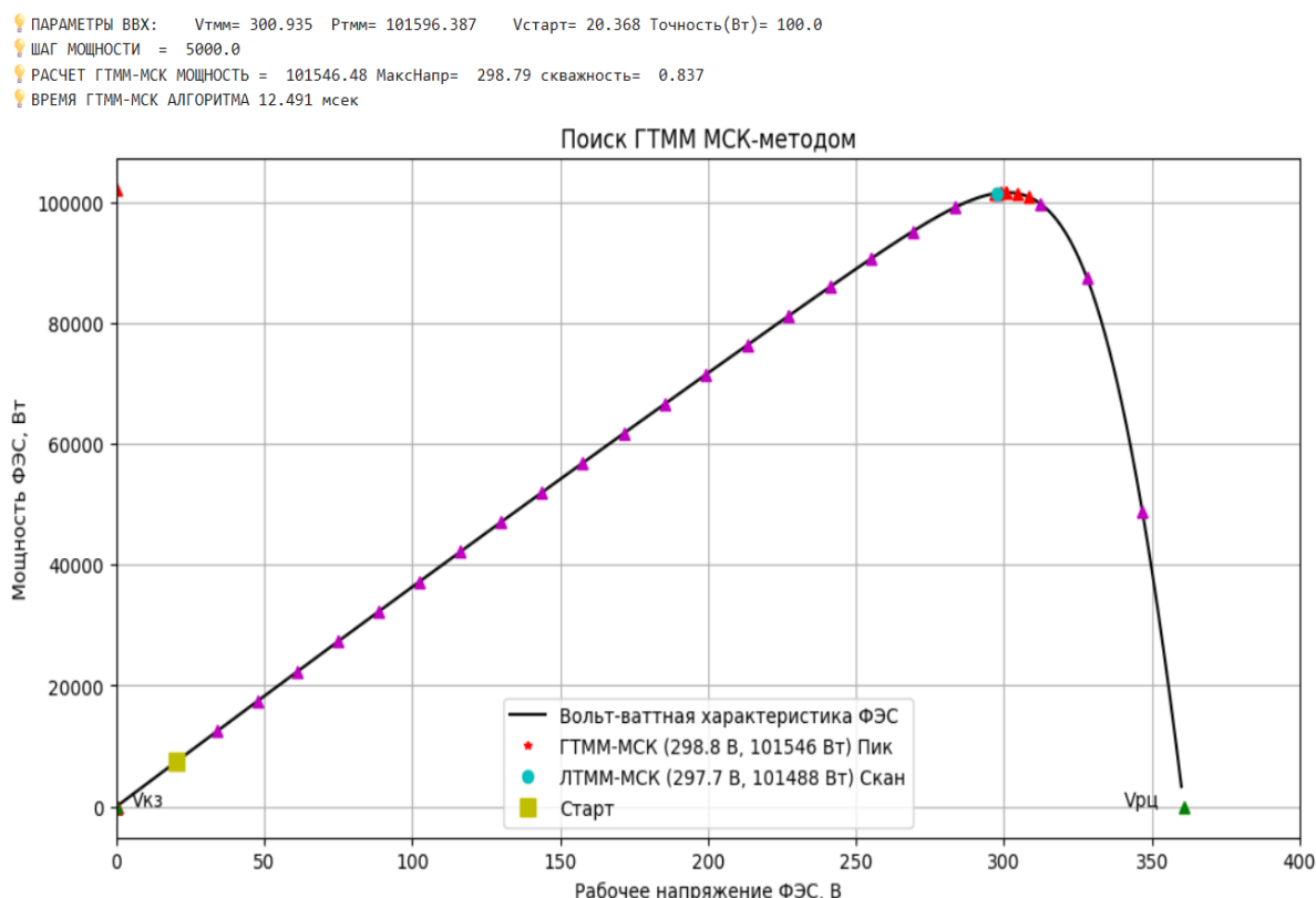
Рисунок 5 – Траектория управления РММ-шаблон 1 с использованием контроллера ГТММ-МСК в Micro-Python
