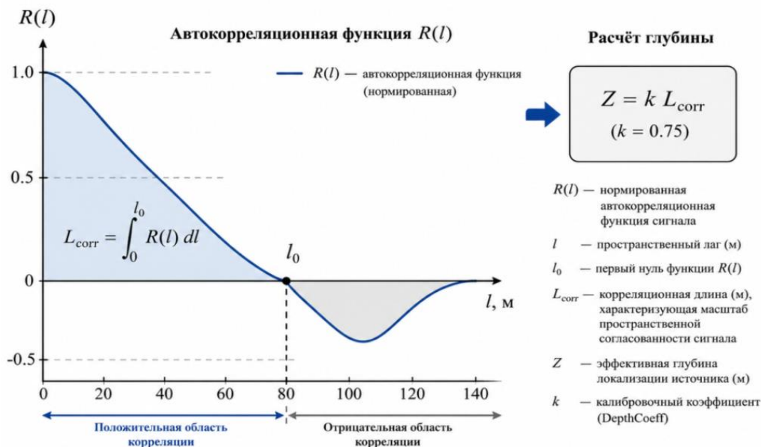
Рисунок 1 – Определение корреляционной длины L_{\text{corr}} по автокорреляционной функции сигнала и её связь с эффективной глубиной локализации источника
