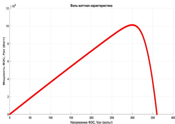
Рисунок 1 – Функция с одним пиком
