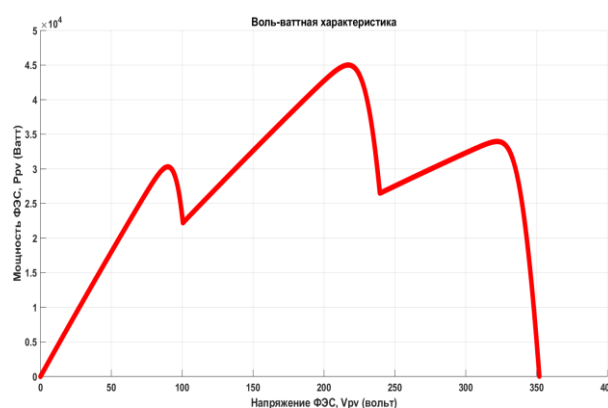
Рисунок 2 – Функция с несколькими пиками
