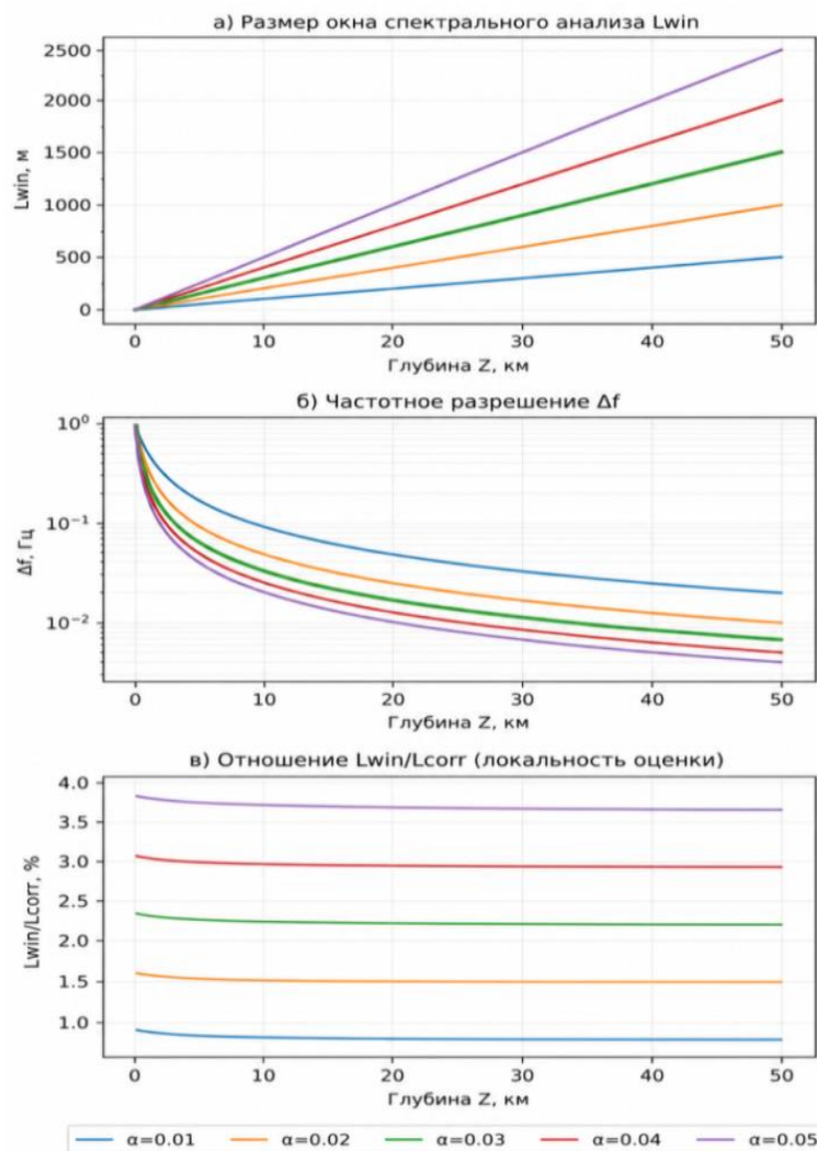
Рисунок 3 – Зависимость параметров спектрального анализа от глубины при различных значениях коэффициента масштабирования \alpha : а) размер окна анализа L_{win} ; б) частотное разрешение \Delta f ; в) отношение L_{win}/L_{corr} , характеризующее локальность оценки.
