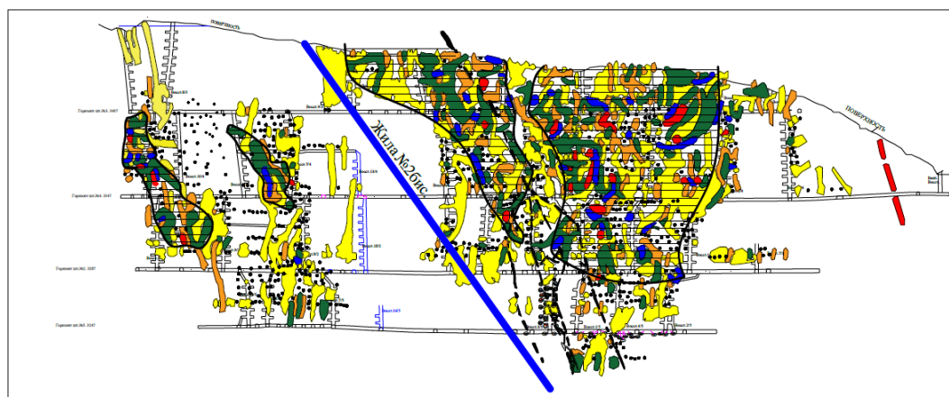
Рисунок 5 – Распределение изоконцентрат классов содержаний золота на продольной проекции рудного тела №2
