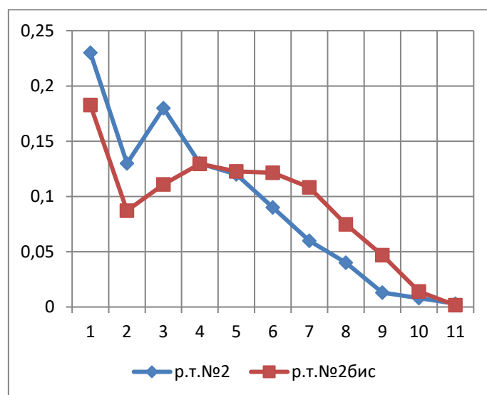
Рисунок 1 – Полигон распределения золота рудных тел №2 и №2 бис
