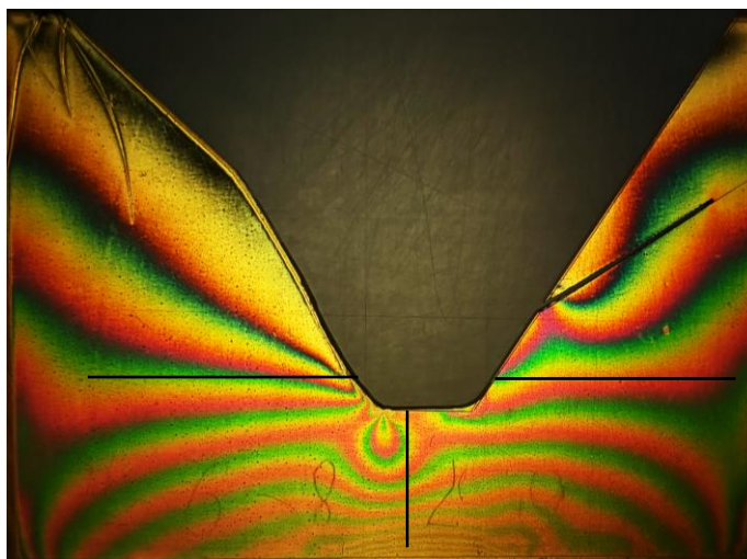
Рисунок 1 - Вид распределения полей напряжений в массиве карьера под влиянием крутопадающего разлома
