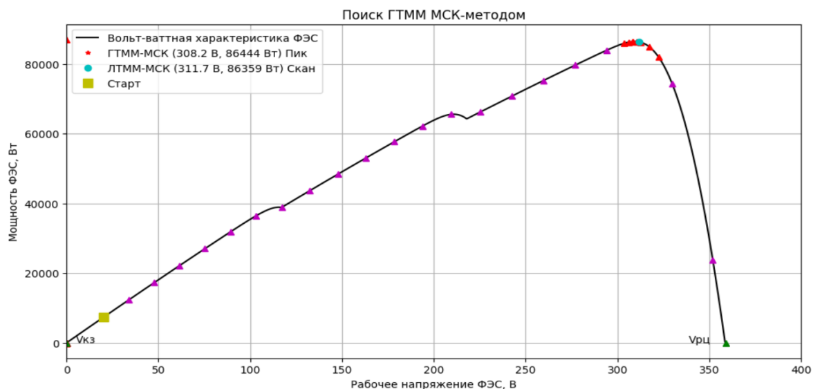
Рисунок 6 –Траектория управления РММ-шаблон 2 с использованием контроллера ГТММ-МСК в Micro-Python
