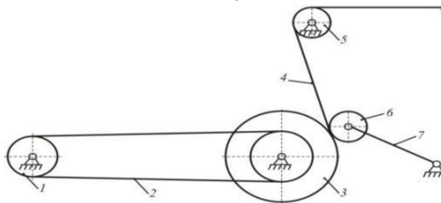
Рисунок 4 – Схема намоточного механизма сновальных машин
