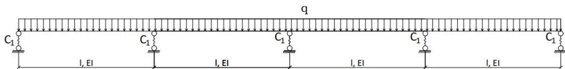
Рисунок 3. Расчетная схема
