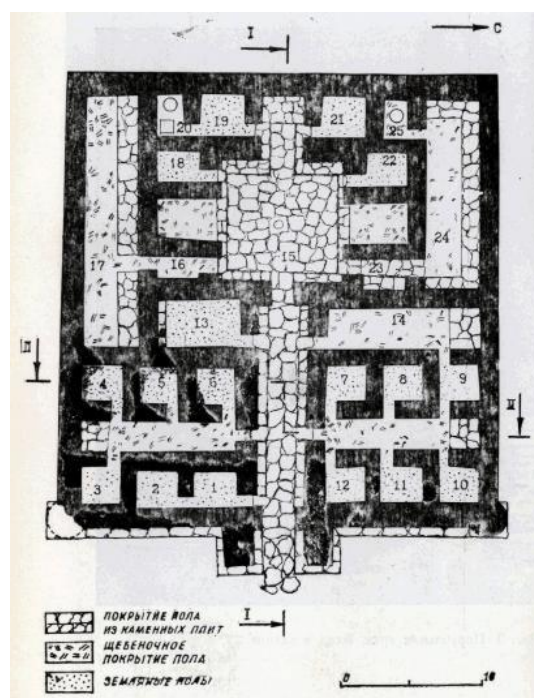
Рисунок 3 – План стен и полов [11]
