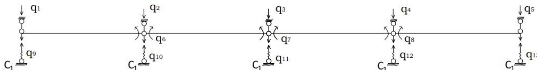
Рисунок 5 – Основная система с конечными элементами второго типа
