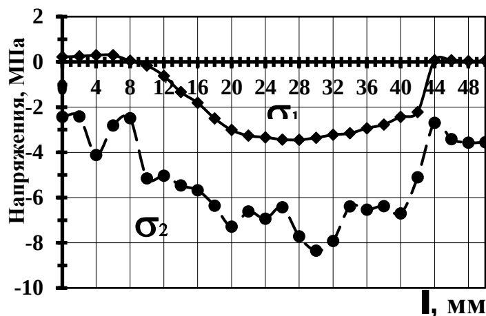
Рисунок 3 - Эпюры главных нормальных напряжений по горизонтальному сечению под разломом на правом борту карьера
