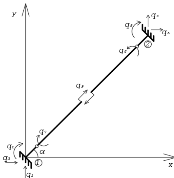
Рисунок 2 – Конечный элемент-стержень смешанного метода
