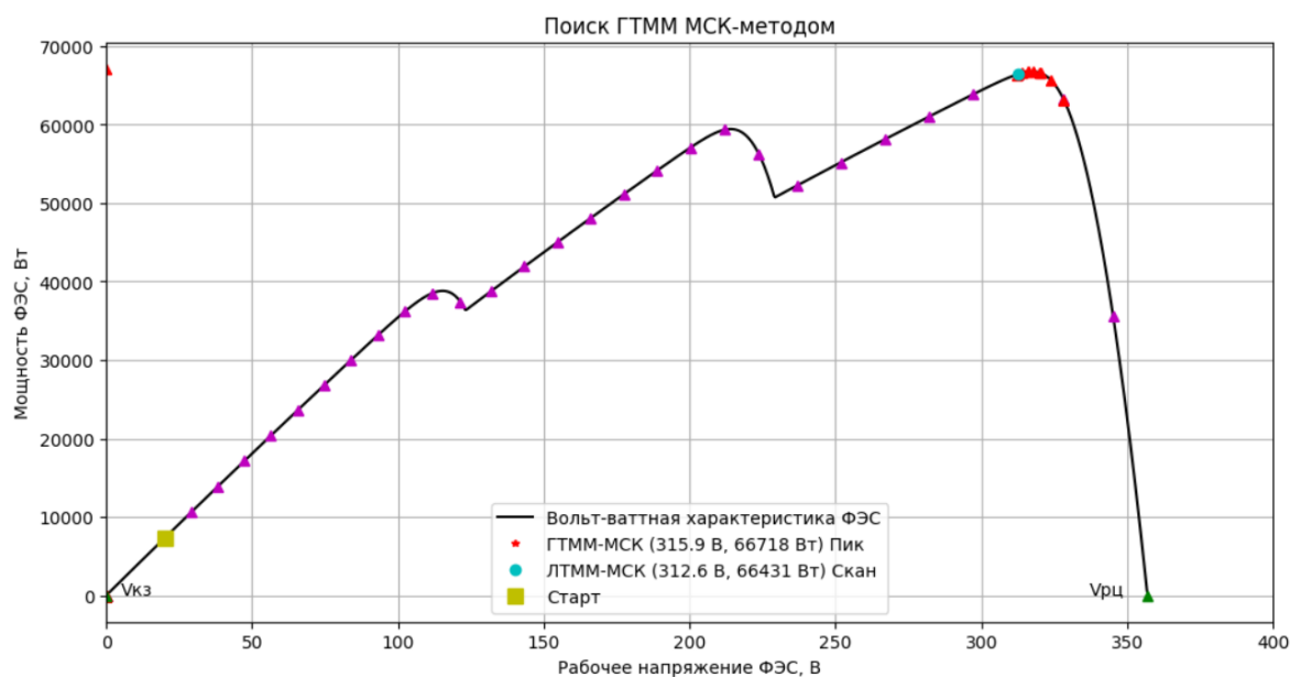
Рисунок 7 –Траектория управления РММ-шаблон 3 с использованием контроллера ГТММ-МСК в Micro-Python
