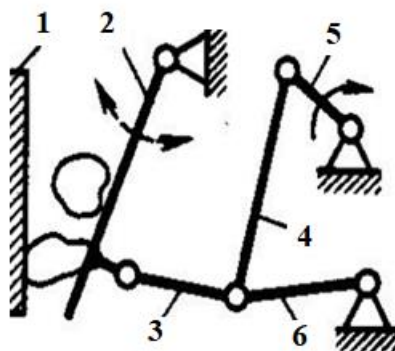
Рисунок 6 – Схема механизма щековой дробилки
