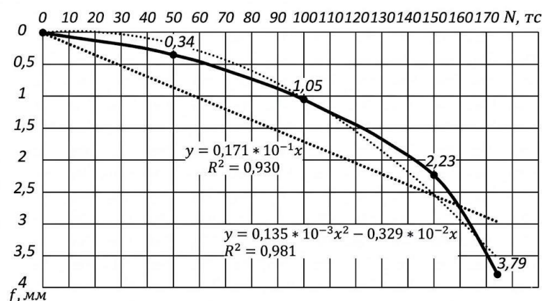
Рисунок 1 – График зависимости осадки сваи от нагрузки
