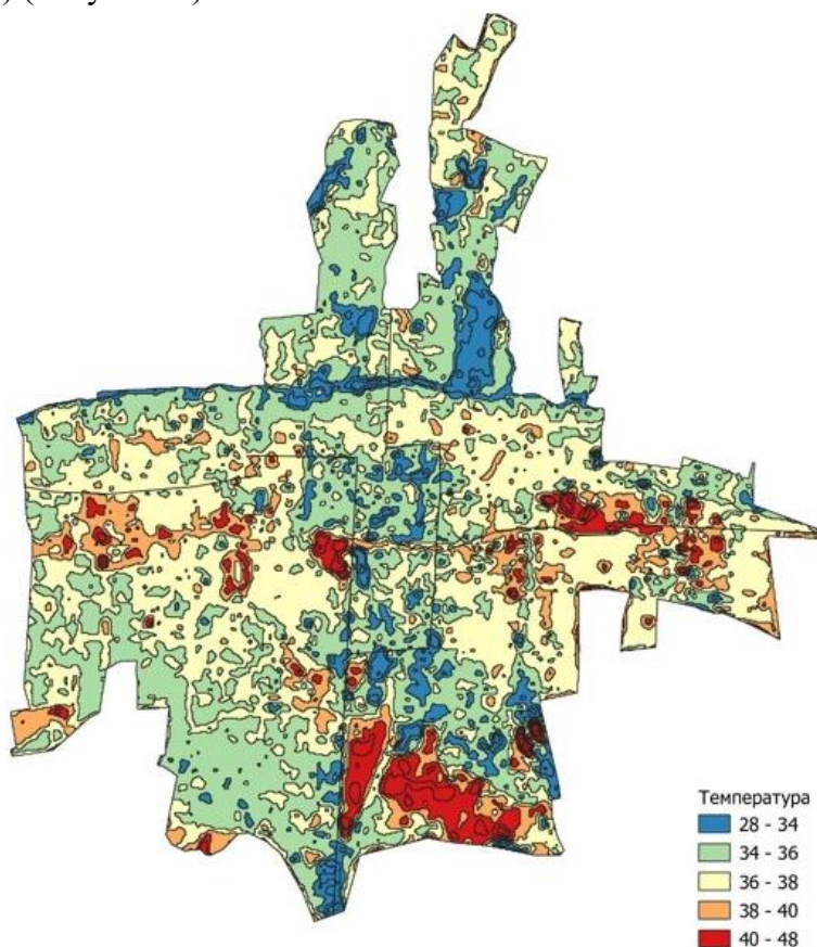
Рисунок 6 – Температура земной поверхности в Бишкеке в жаркий летний день (данные спутникового тепловизора): зелёным/синим показаны более прохладные районы (парки, водоёмы, пригороды с растительностью, температура ~28-34 °C), жёлтым/оранжевым – нагретые территории (плотно застроенные кварталы, 36-40 °C), красным – наиболее горячие «пятна» (до +48 °C на солнце) в промзонах и новых микрорайонах с отсутствием озеленения.
