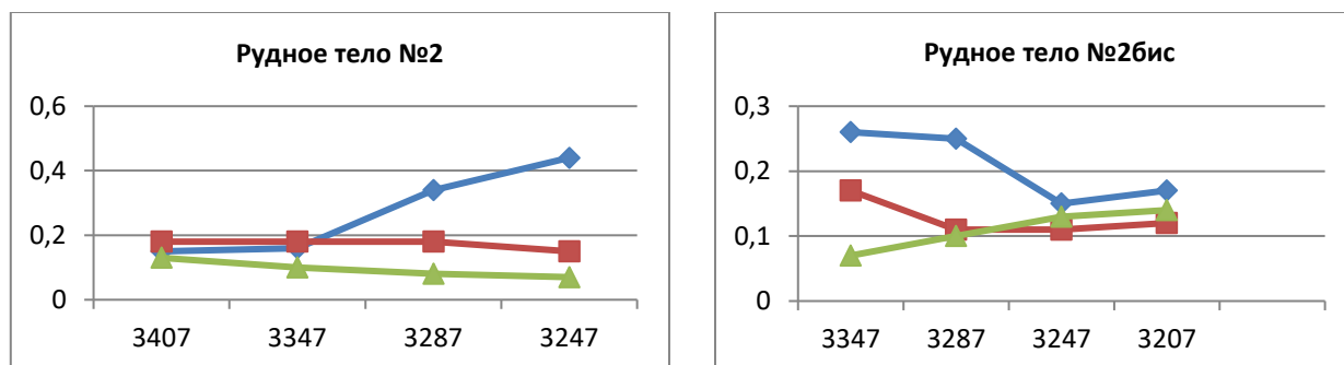
Рисунок 3 – Изменение мод 1,3,6 по падению рудных тел №2 и №2бис, условные
