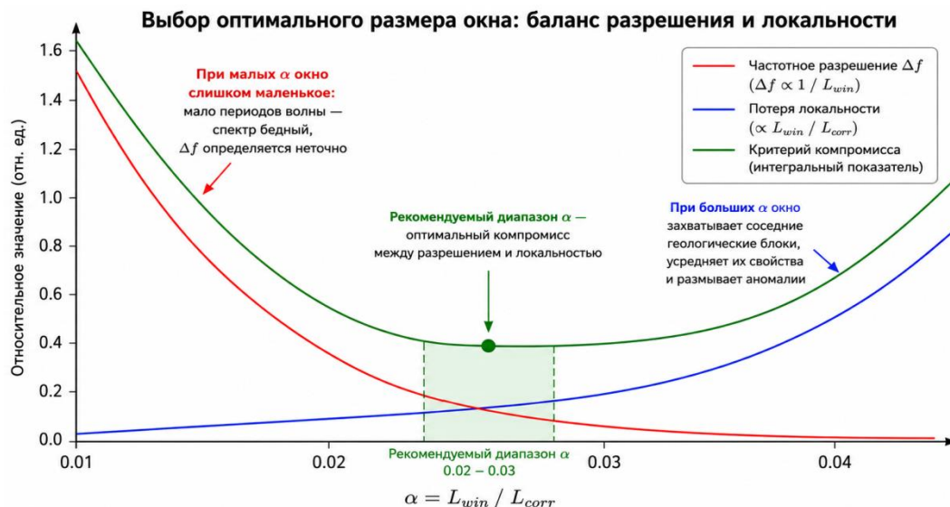
Рисунок 2 – Изменение частотного разрешения и пространственной локальности в зависимости от относительного размера окна анализа
