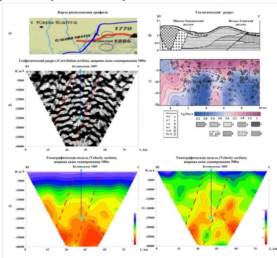
Рисунок 4 – Сопоставление томографических моделей GPTS с данными магнитотеллурического зондирования (МТЗ) вдоль профиля, пересекающего Шамсин-Тюндюкский и Иссык-Атинский разломы: а — карта расположения профиля; б —
