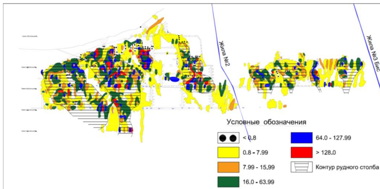
Рисунок 6 – Распределение изоконцентрат классов содержаний золота на продольной проекции рудного тела №2 бис
