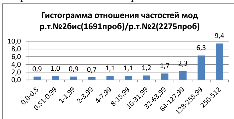
Рисунок 4 – Кратность представительности вероятности проявления классов содержаний в рудных телах(частное частоты классов р.т.№2бис к р.т.№2)
