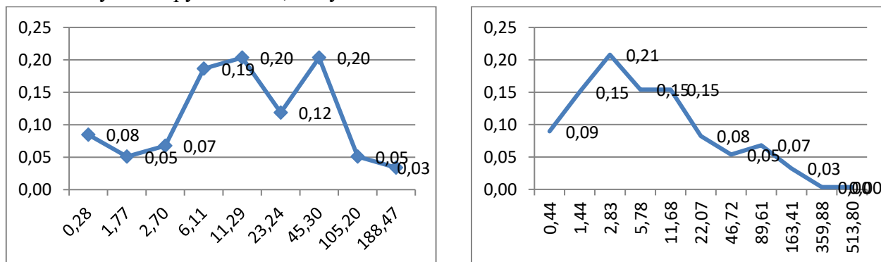
Рисунок 2 – Иллюстрация полимодальности рудных тел №2бис(слева- блок 5-13C1.) и №2(справа- блок 4-2C1.) по разведочно-эксплуатационным блокам(выборки более 200)
