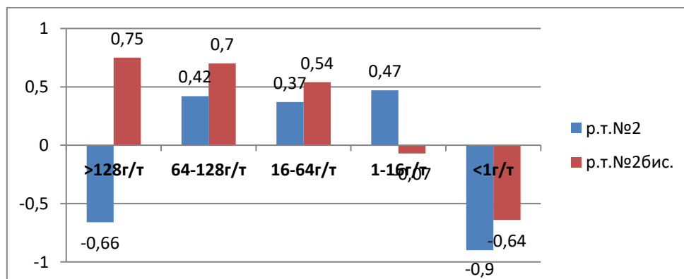
Рисунок 7. – Ранговая корреляция классов золота рудных тел №2(1182наблюдения), №2бис (992 наблюдения)
