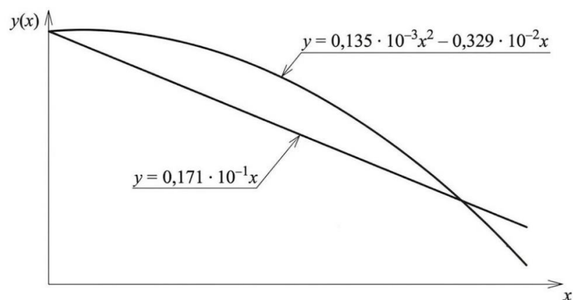
Рисунок 4 – График описывающий жесткость свай
