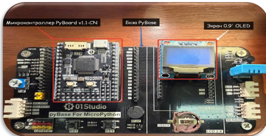
Рисунок 3 – Внешний вид программируемой платформы PyBoard с микроконтроллером STM32
