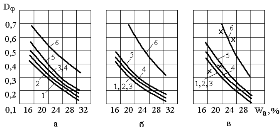
Рис. 2. Зависимость динамического фактора по сцеплению D_\phi от влажности грунтов: а – легкий суглинок; б – средний суглинок; в – тяжелый суглинок. Автомобили: 1 – ГАЗ-52-03; 2 – ГАЗ-53А; 3 – ЗИЛ-130; 4 – КамАЗ-5320; 5 – Урал-377; 6 – Урал – 5557.
