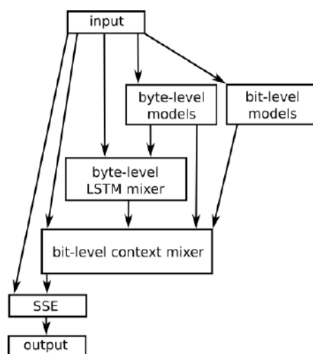
Рис. 2. Архитектура cmix
