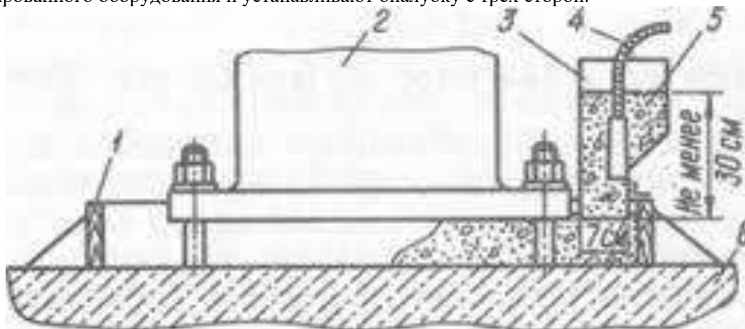
Рис.1. Бетонирование полости под промышленным оборудованием с применением метода механического зачеканивания: 1 - опалубка; 2 - оборудование; 3 - подливочная смесь; 5 -фундамент; 4 - ручной инструмент
