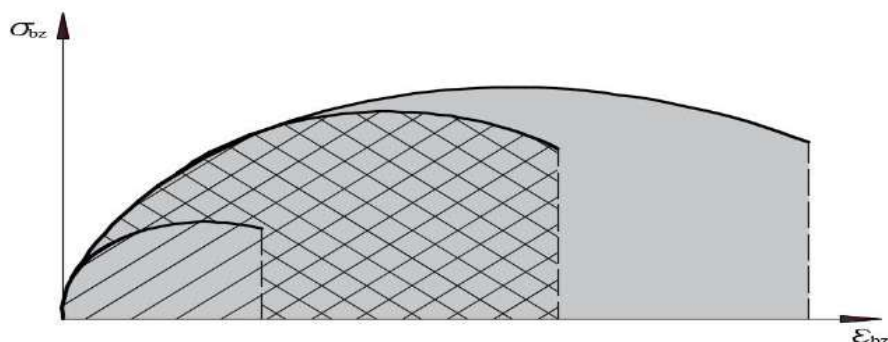
Рис. 6. - - работа, которую нужно потратить на разрушение железобетонной колонны - работа, которую нужно потратить на разрушение сталетрубобетонной колонны - работа, которую нужно потратить на разрушение сталетрубобетонной колонны со спиральным армированием
