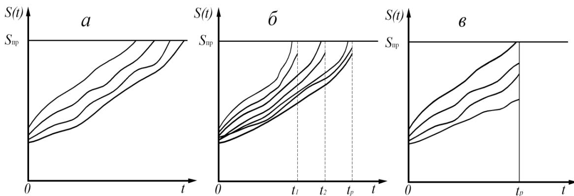
Рис. 1. Стратегии обеспечения работоспособности изделий: а – эксплуатация до наступления отказа; б – по состоянию с контролем параметров; в – по назначенной наработке; t_p – наработка изделия до ремонта; t_1, t_2, t_3 – наработки до проведения контрольно-диагностических операций
