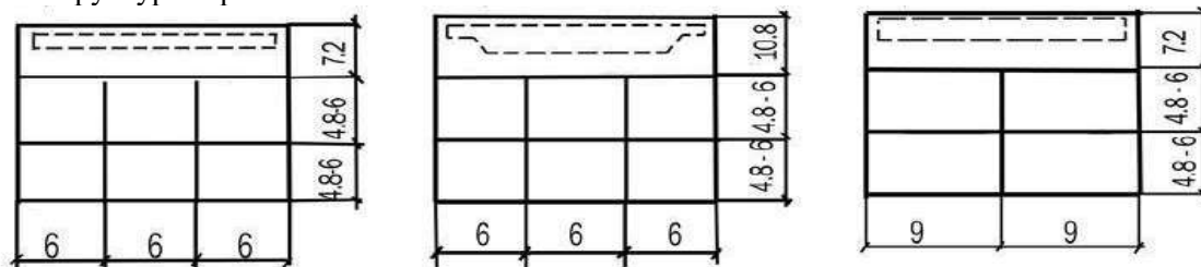
Рис. 4. Унифицированные габаритные схемы многоэтажных зданий
