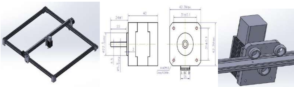
Рис. 1. 3D модели лазерного станка
